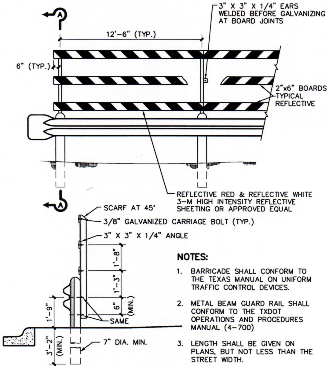
SECTION A-A
